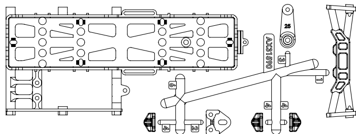
AX31590 (x1) Battery Tray and Servo Mount Set Akkualterung- und Servohalterungssatz Ensemble de supports de servo et support de batterie Set vassoio portabatteria e supporti servo
