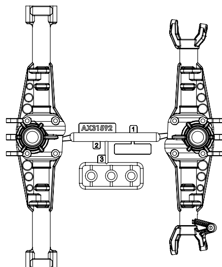
AX31592 (x1) AR44 Solid axle housing, front and rear AR44 solides Achsgehäuse, vorne und hinten Carter d'essieu solide AR44, avant et arrière Alloggiamento solido assale AR44, anteriore e posteriore
