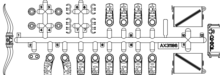
AX31186 (x3) M4 Rod End Set M4 Stangenkopfsatz Ensemble d'embout de bielle M4 Set teste a snodo M4
